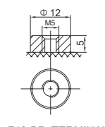
F13-BP TERMINAL
